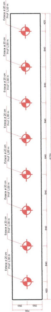
PLANTA BAIXA LOCAÇÃO ESTACAS
