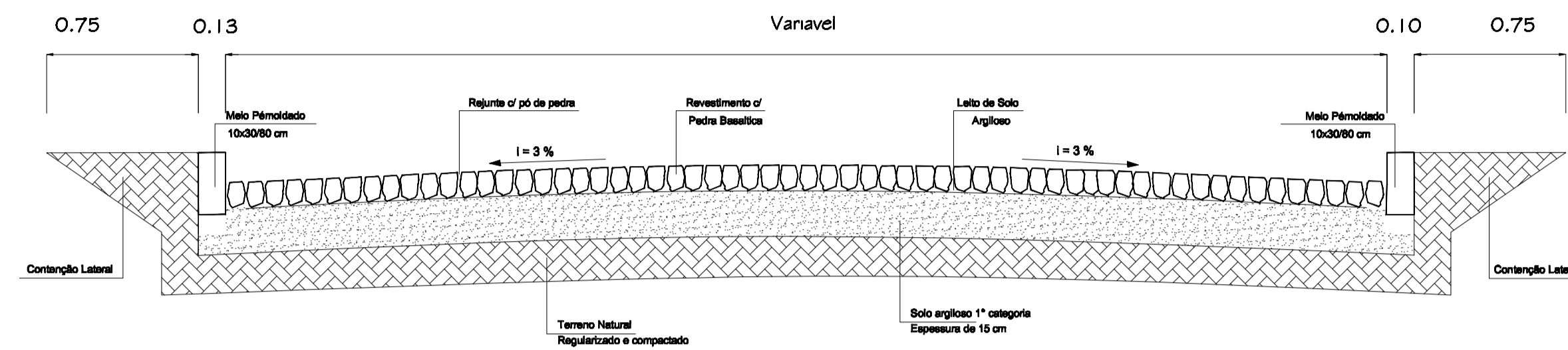
SEÇÃO TRANSVERSAL TIPO SEM ESCALA
