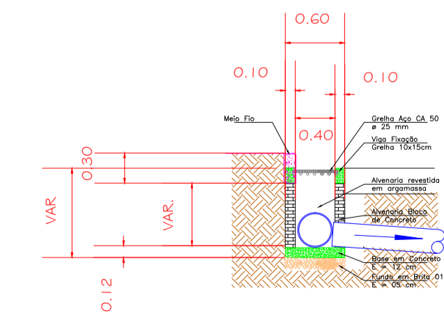
CORTE ESC. 1:50
