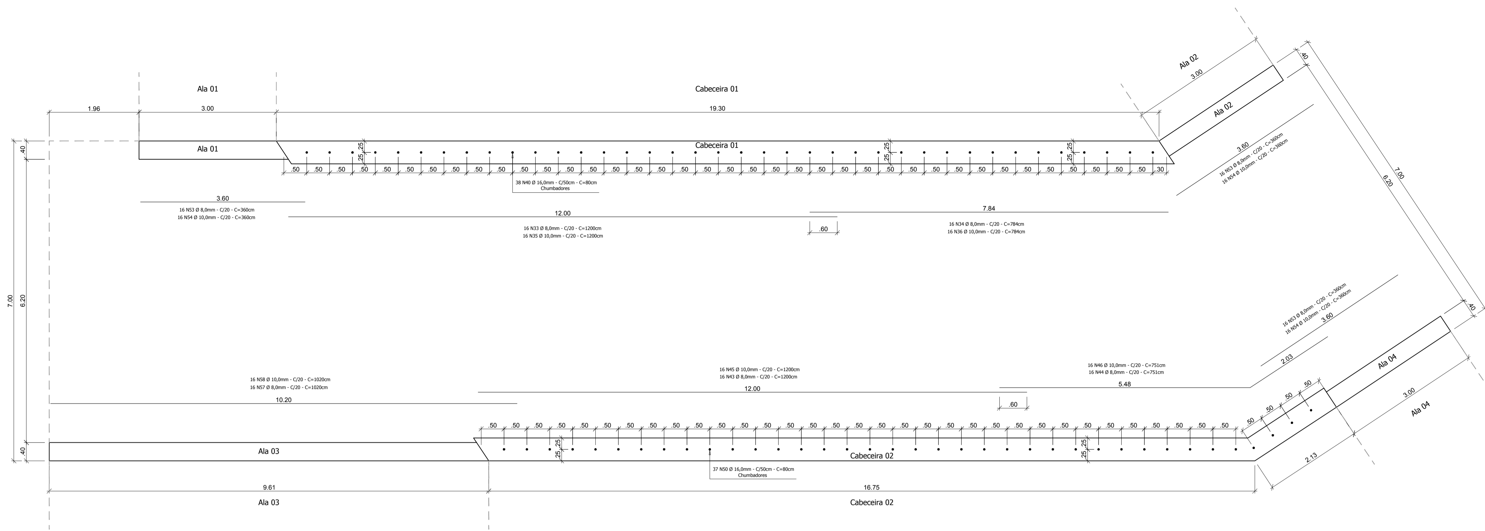
Vista Superior das Cabeceiras / Alas esc. 1/50
