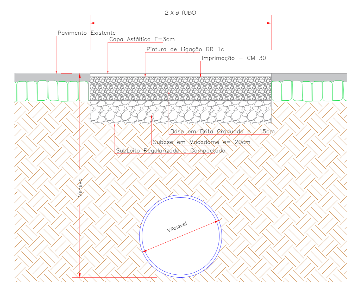
CORTE BL/01-130x80/120 ESC. 1:25
