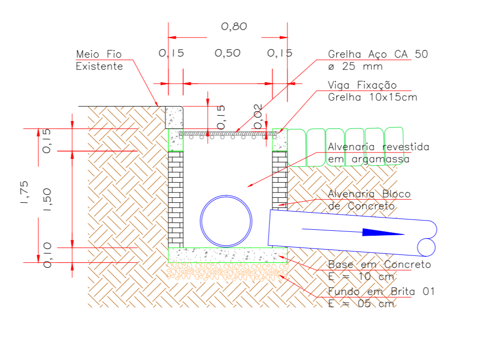
CORTE BL/01-130x80/120 ESC. 1:25
