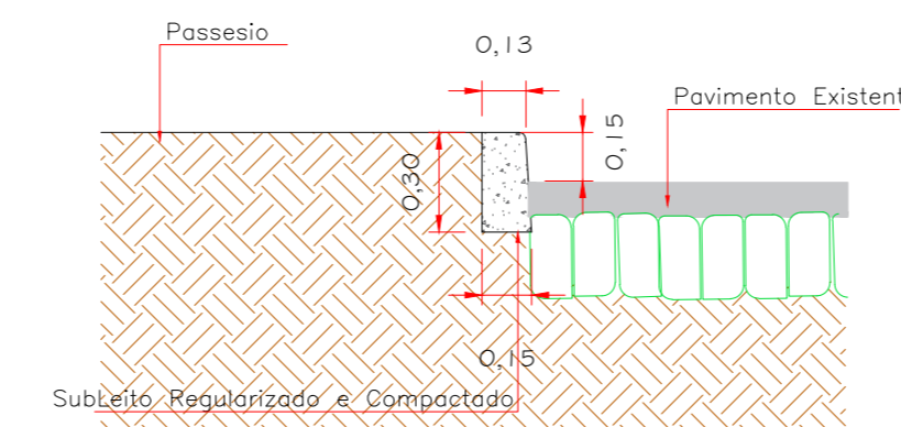
CORTE MEIO FIO PRÉ-MOLDADO ESC. 1:25
