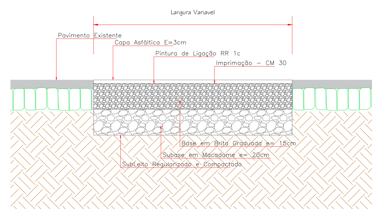
CORTE REMENDO PROFUNDO ESC. 1:25
