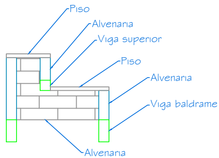
DETALHE escala 1:50
