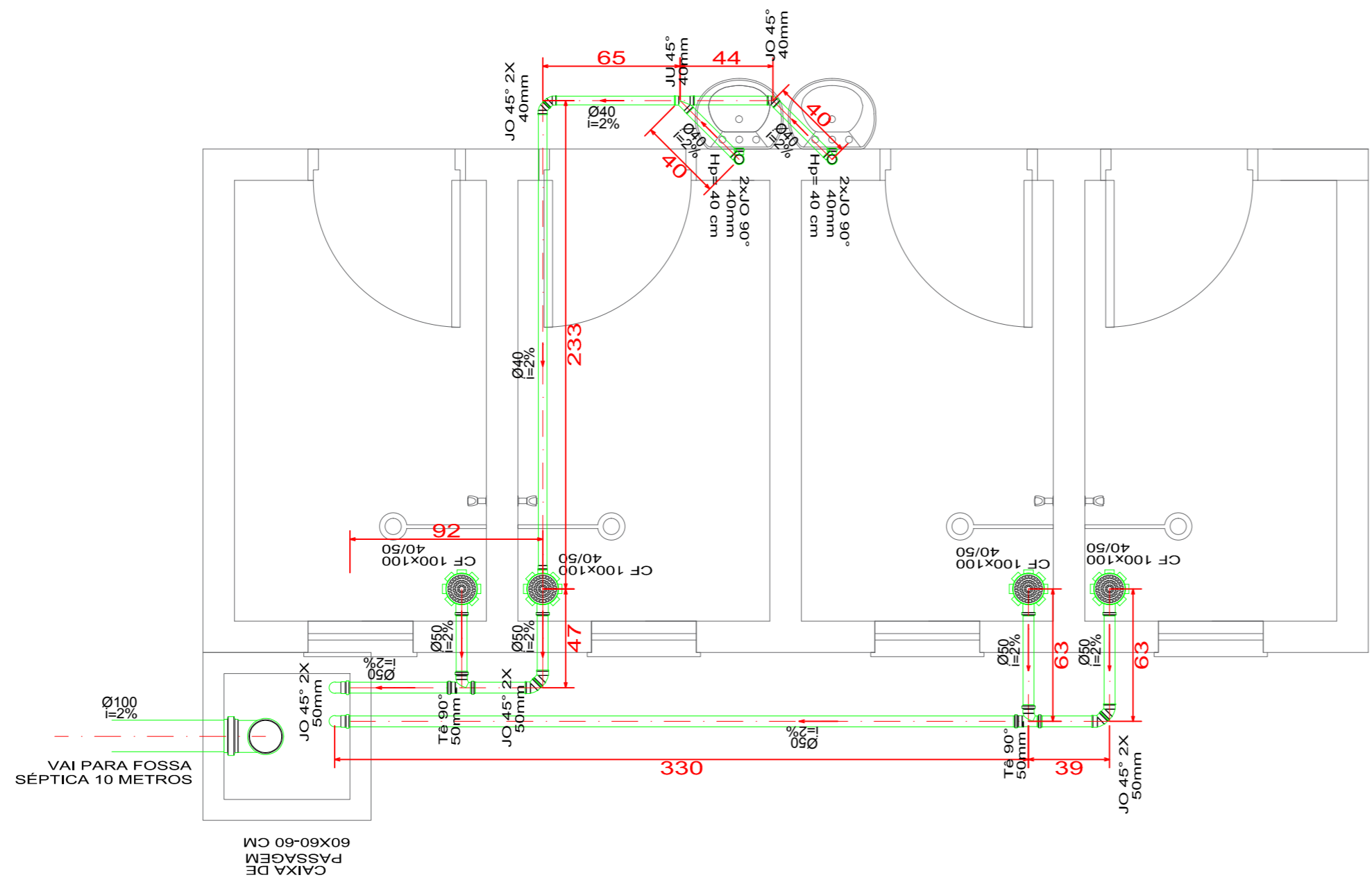
Planta Baixa – Esgoto Escala 1:25
