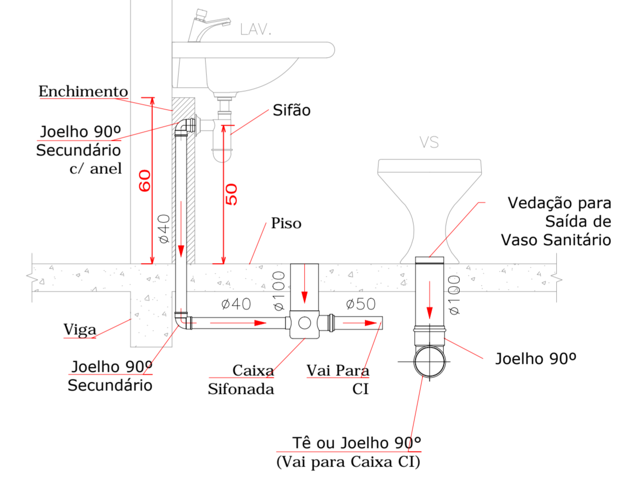
DETALHES LIGAÇÕES
