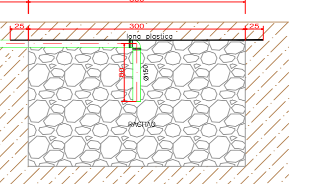
Corte AA – Sumidouro Escala 1:50
