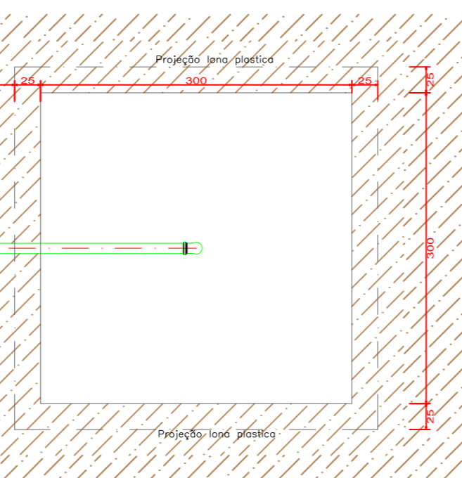
Planta Baixa – Sumidouro Escala 1:50
