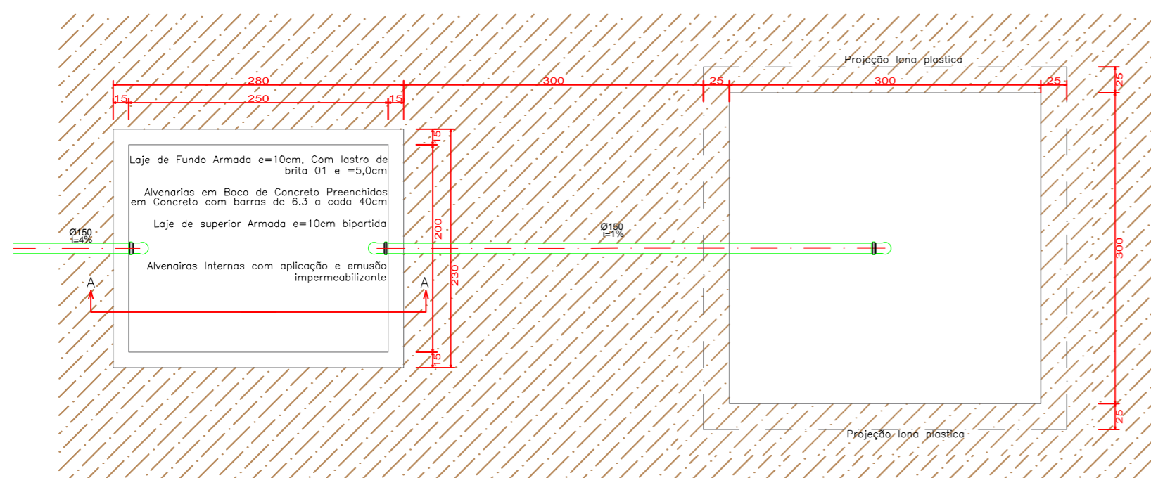
Planta Baixa – Fossa Séptica Escala 1:50
