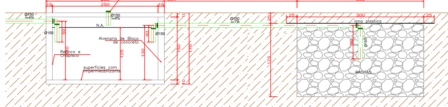
Corte AA – Fossa Séptica Escala 1:50
